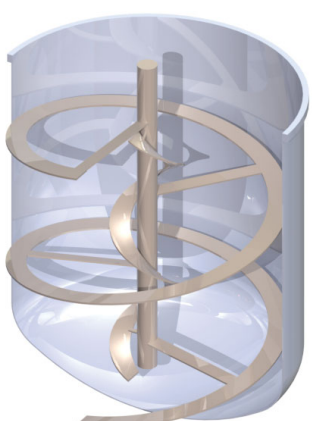
Áncora tipo helicoidal
