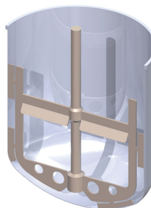
Áncora en "U" con pala
